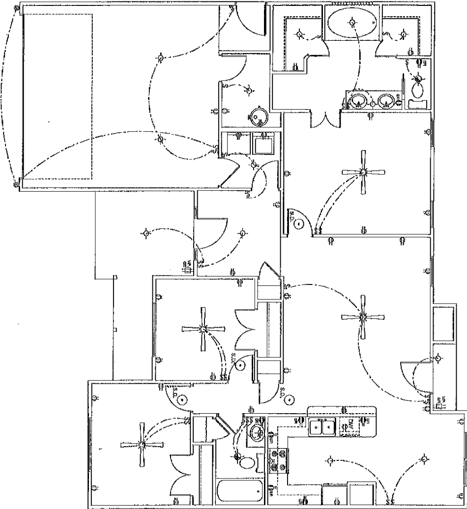
ELECTRICAL PLAN SCALE: 1/8" = 1'-0"
